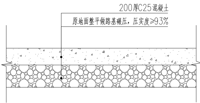
车行便道路面做法 1:20
